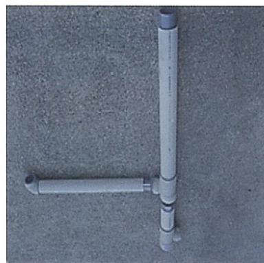
直管寸法切り+継手ユニット (3パーツ)
