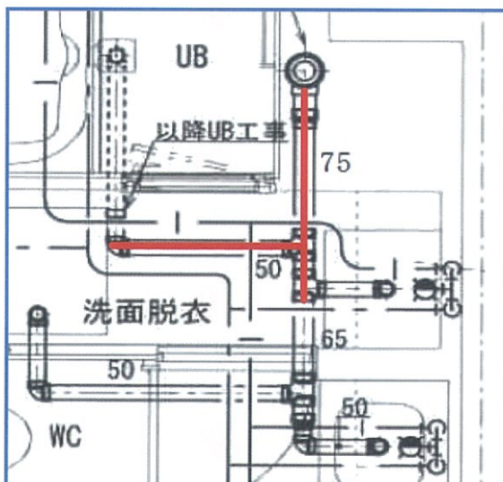
横枝管ユニット
